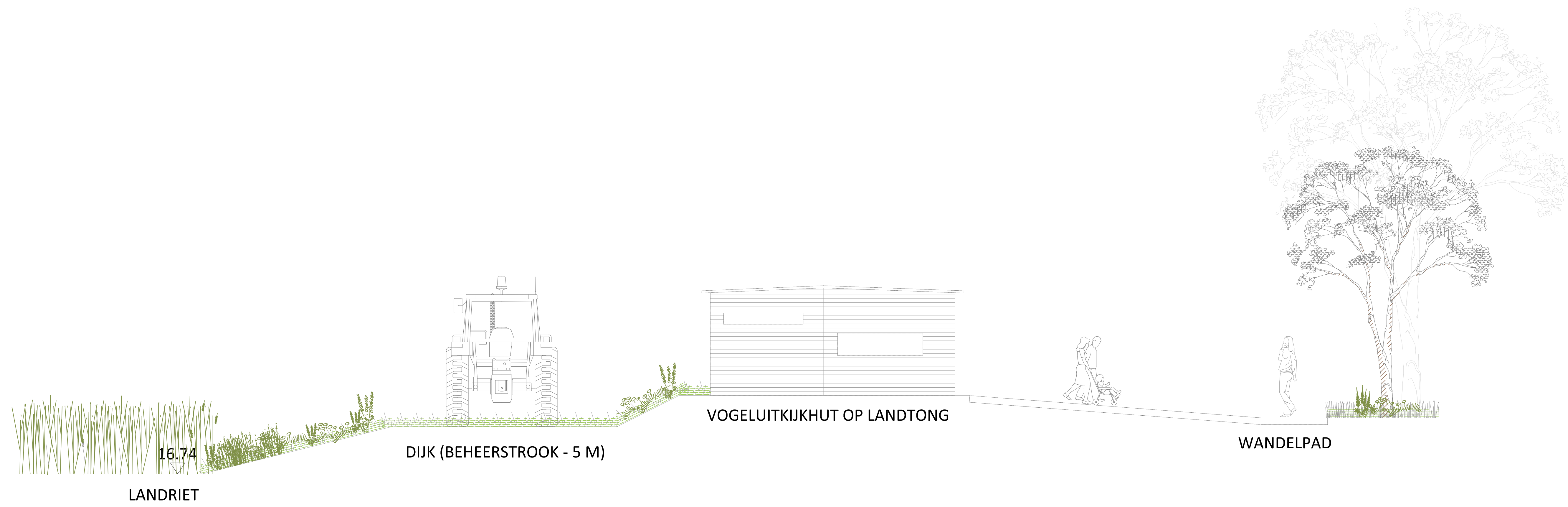
Doorsnede ter hoogte van nieuwe vogelkijkhut
