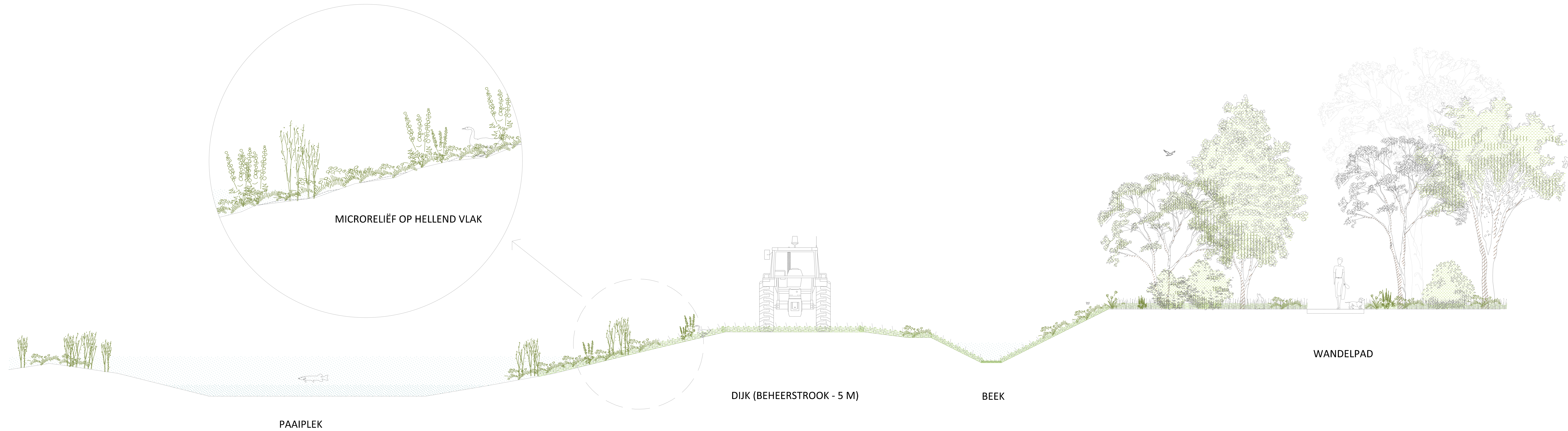
Doorsnede vijver en nieuwe bedding Spoelbeek met tussenin een onderhoudsdijk
